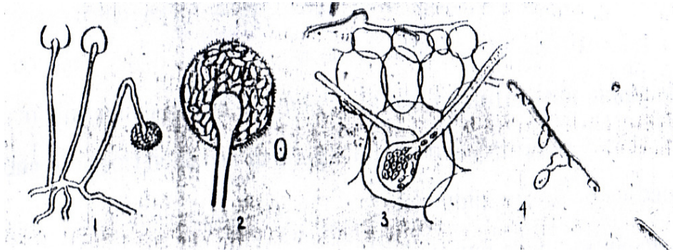
Hình 3: Bọc và bọc bào tử động
